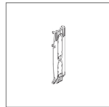
Kabelová příchytka bezhalogenový PC-ABS
