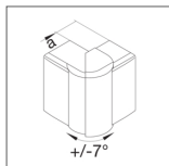
Vnější roh nastavitelný bezhalogenový PC-ABS ABS
