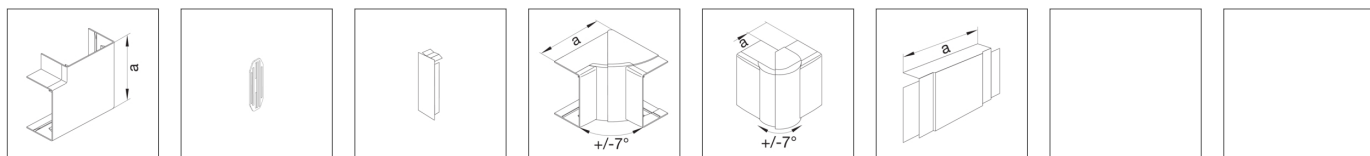
Spojka bezhalogenový PC-ABS Koncový díl ABS Vnitřní roh nastavitelný bezhalogenový PC-ABS Vnější roh nastavitelný bezhalogenový PC-ABS T- a křížový kus bezhalogenový PC-ABS Kryt řezu ABS Kabelová přichytka bezhalogenový PC-ABS
